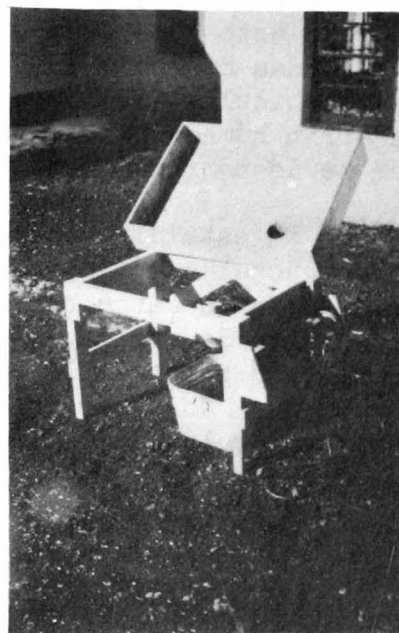
Mezclador de ventilador usado en la preparación de mezclas de carne y forraje seco.
