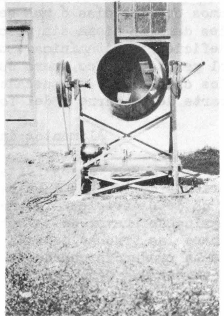
Mezcladora para dietas de carne y forraje seco.
